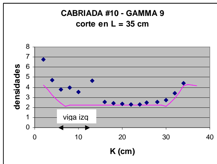
Figura 14. Densidades medidas (puntos azules) y fondo calculado (línea magenta), para la gammagrafía 9 en un corte para L = 35 cm (atravesando las 3 vigas).
