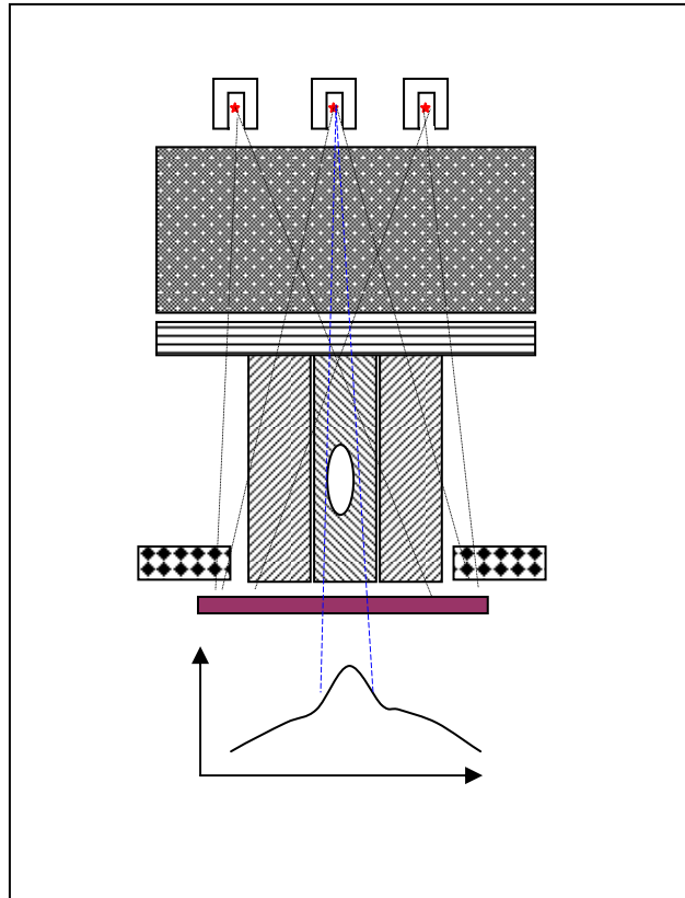
Figura 8. Esquema ilustrativo de mediciones realizadas en cada sector de punto tangente. Los bloques sombreados representan, de arriba a abajo, las tejas, los tabloncillos y las cabriadas.
